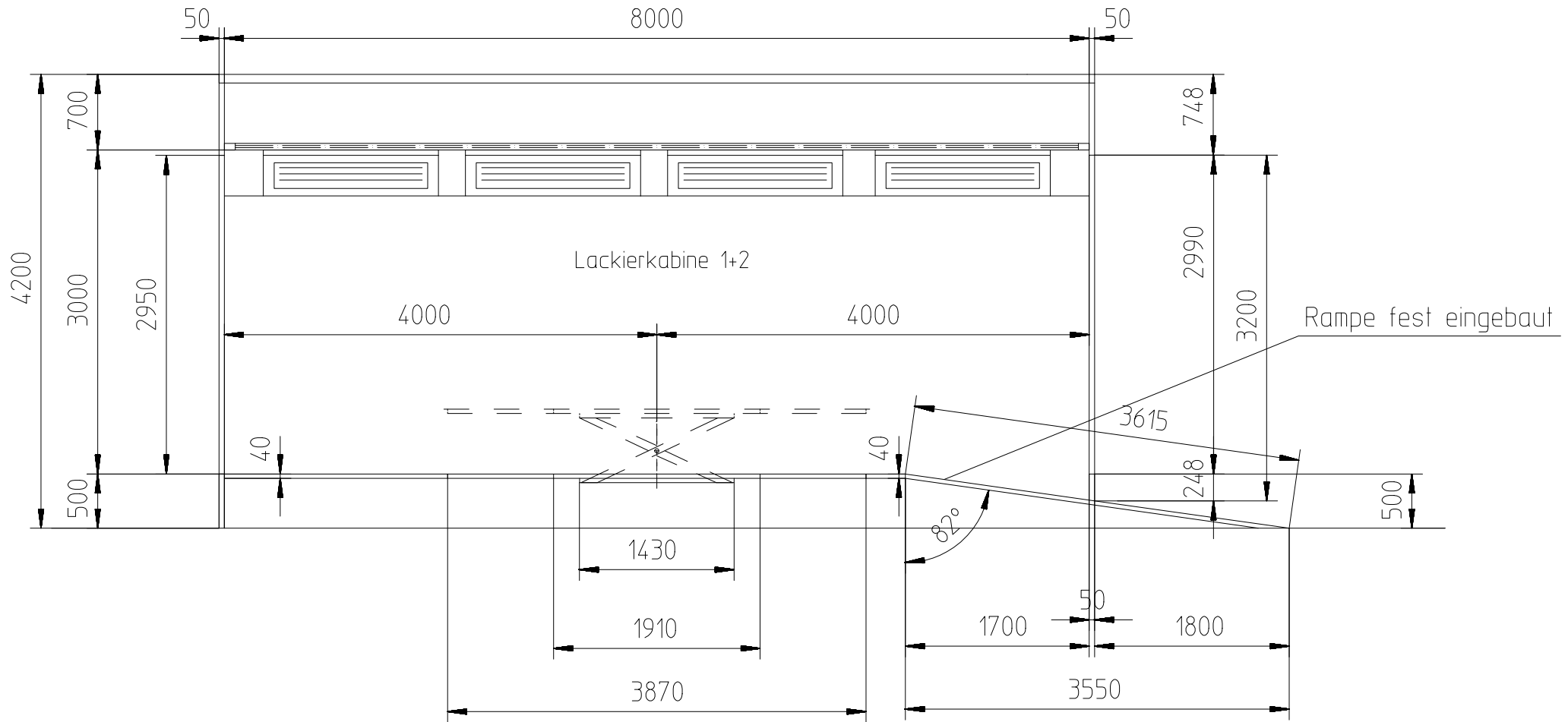
Harper-Detail Rampe / Änderung vom 26-09-2013
